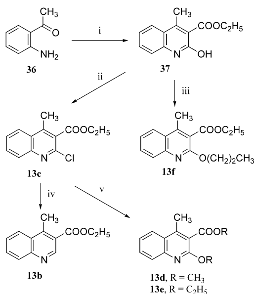
Scheme 8. Reagents: (i) (a) \text{ClCOCH}_2\text{COOC}_2\text{H}_5 , \text{CH}_2\text{Cl}_2 ; (b) \text{NaH} , \text{EtOH} ; (ii) \text{POCl}_3 ; (iii) (a) \text{NaH} , \text{DMF} ; (b) \text{CH}_3(\text{CH}_2)_2\text{I} ; (iv) \text{H}_2 (14 psi), \text{Pd/C} , \text{Et}_3\text{N} , \text{EtOH} ; (v) \text{NaH} , \text{ROH} .
